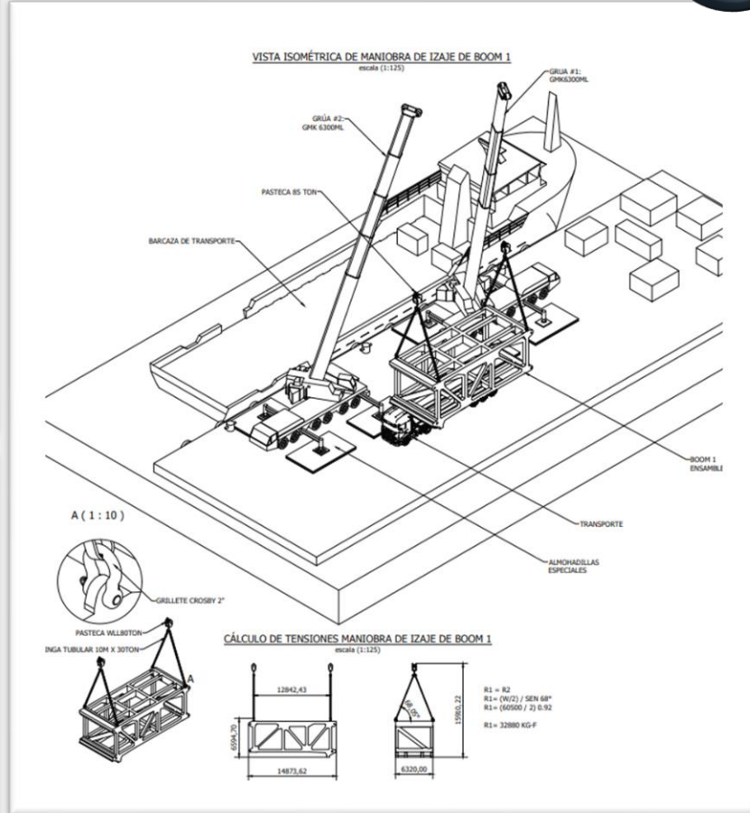
Simulación 3D – Diagrama Izaje BOOM 1
