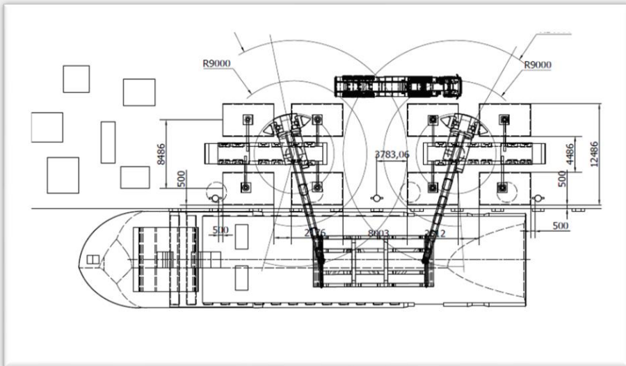
Planes de Trinca y Estiba – BOOM 1
